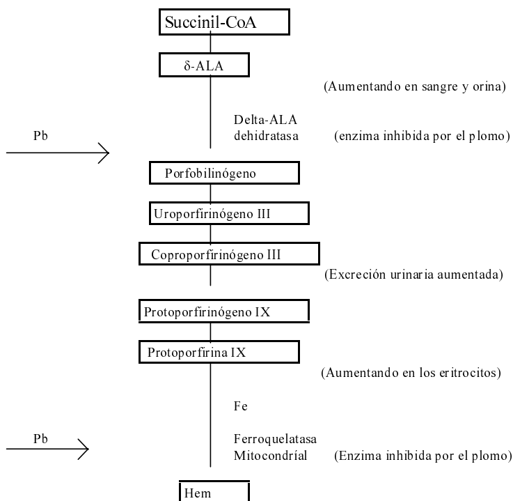
Figura 2. Efectos del plomo en la biosíntesis del Hem (Ellenhorn, 1988)
